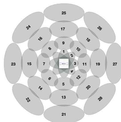
Vue inférieure des 28 faisceaux
